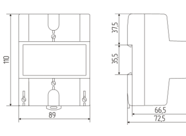
Рисунок А.4 – Габаритные и установочные размеры счетчика CE 200 R5
