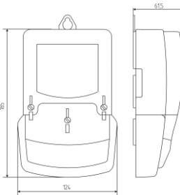
Рисунок А.3 – Габаритные и установочные размеры счетчика CE 200 S10
